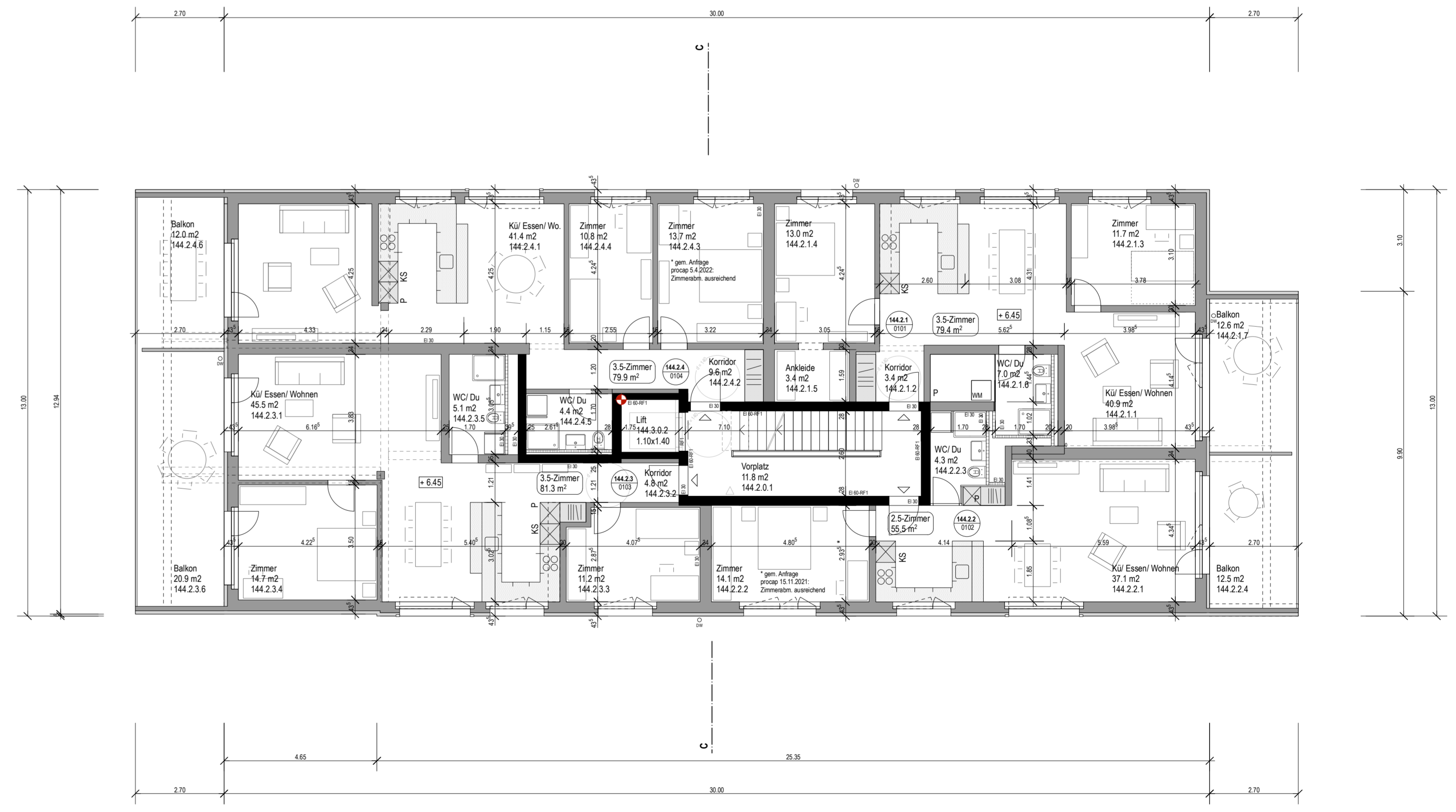
1. OG
