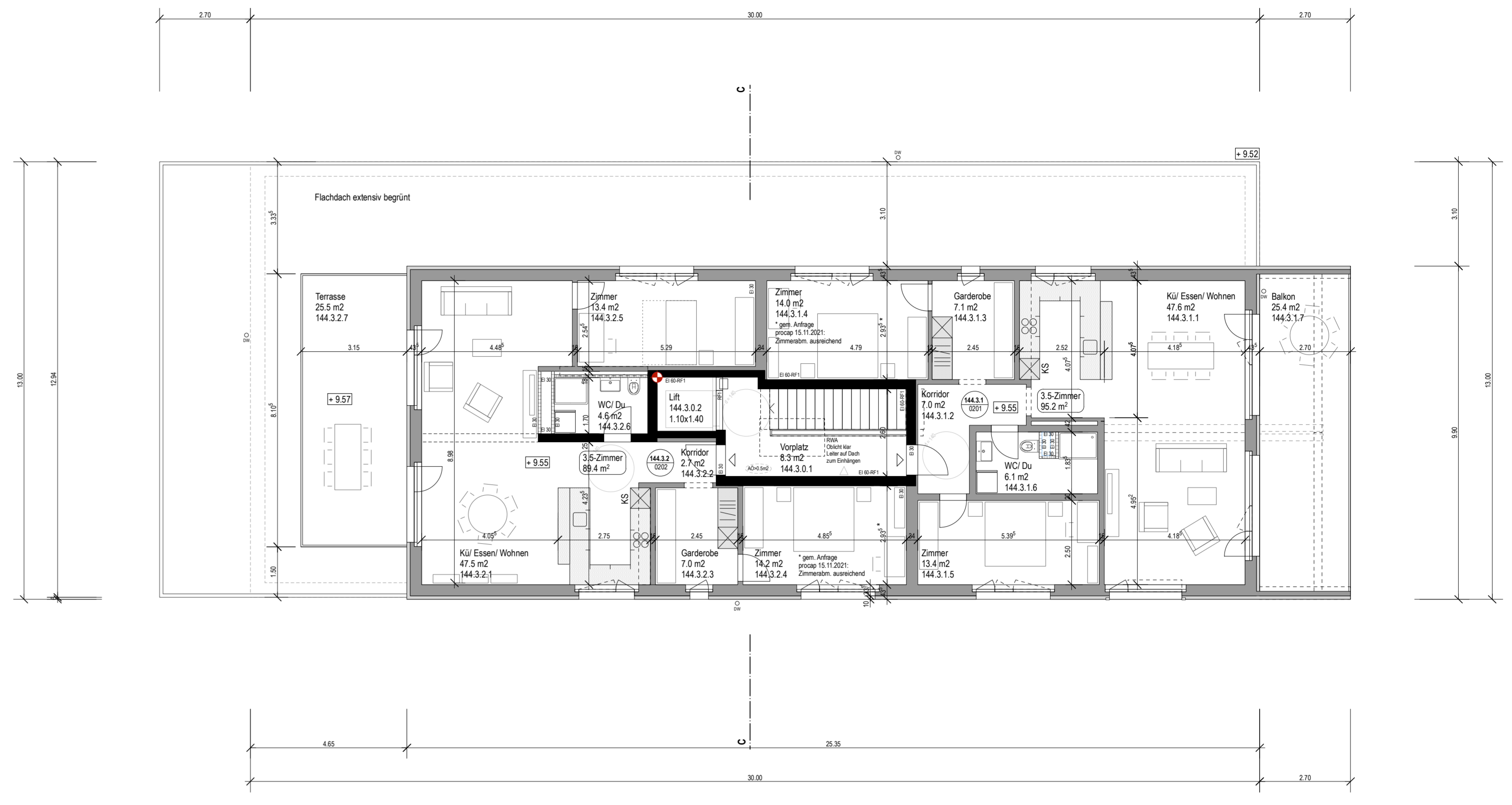
2. OG - Attika
